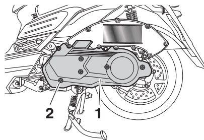
1. V型皮帶箱空氣濾清器蓋 2. 螺栓(x6)
