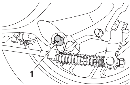
1. 排油螺栓
